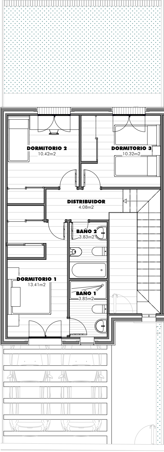
02 PLANTA PRIMERA
