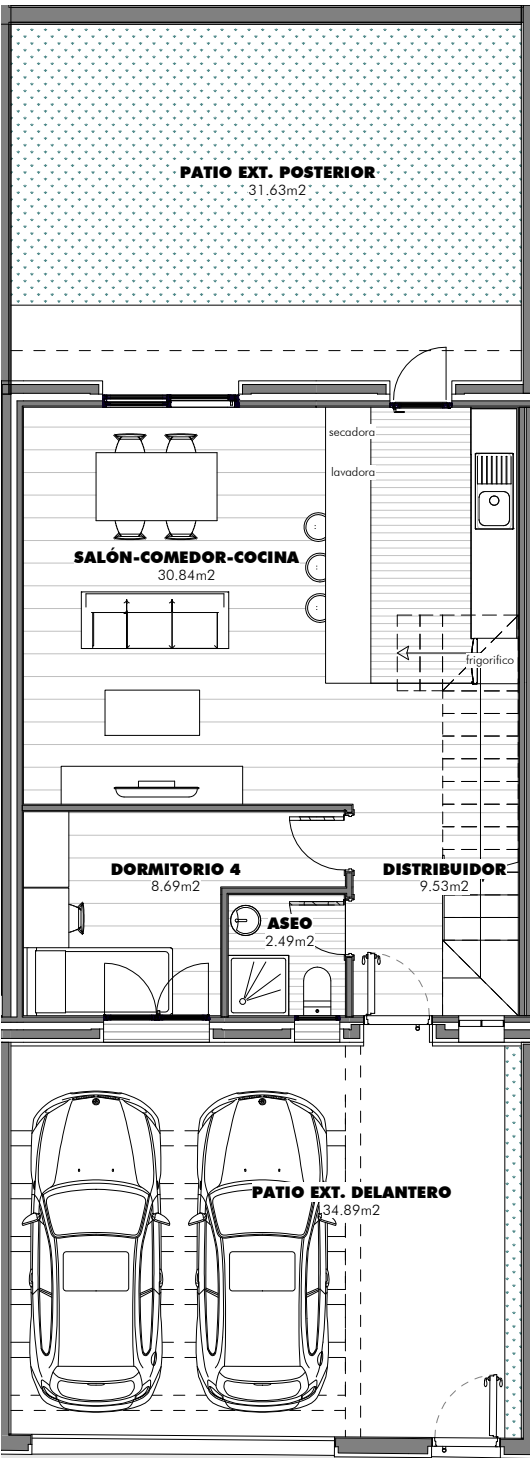
01 PLANTA BAJA
